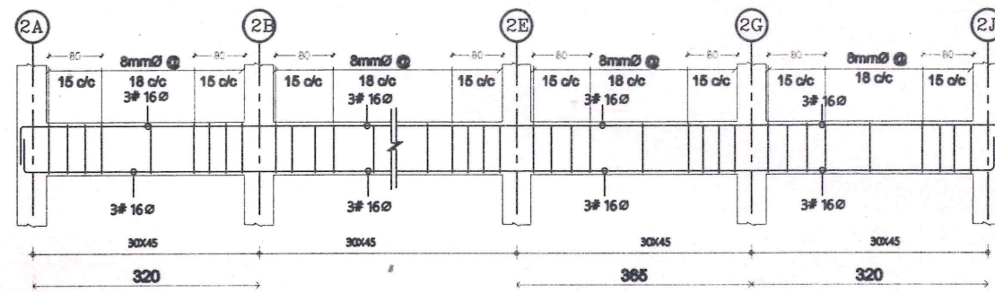
BEAM FB6 (2A-2J)
